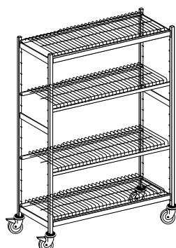
Mobil hyllställning med 4 st trådgallerhyllor.
